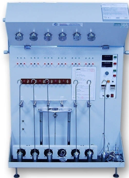
Plug Impact Tester 插頭突拉測試
