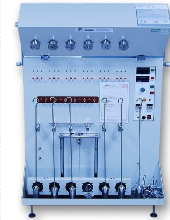
Plug Impact Tester 插頭突拉測試
